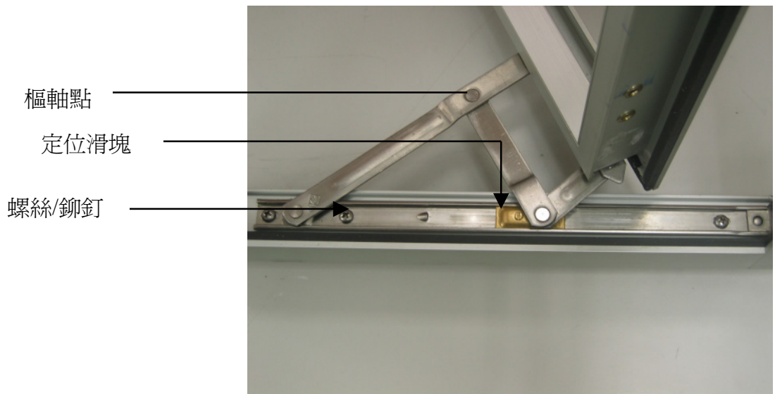
4 桿形窗鉸的構件
